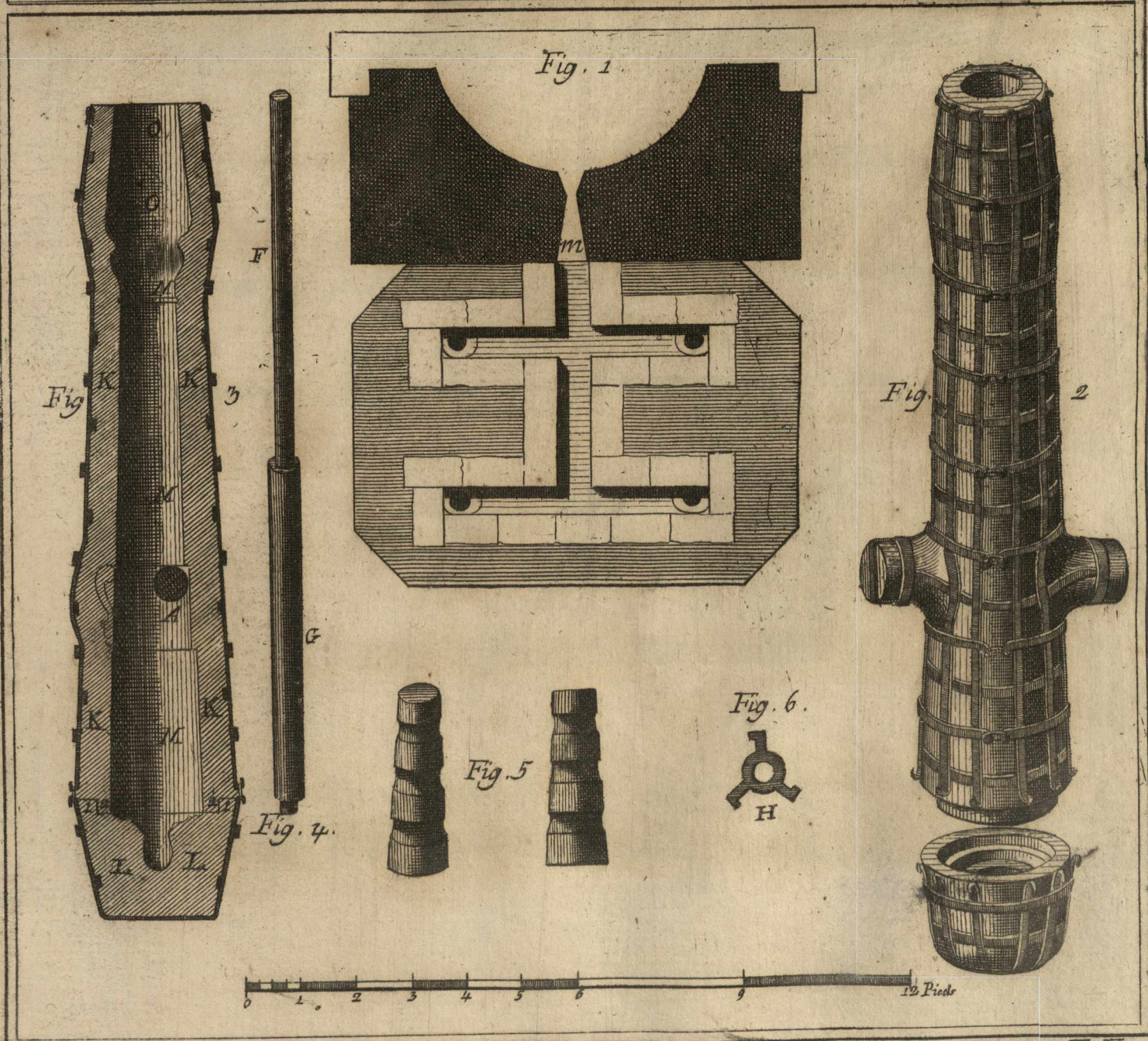
Fonte des Canons, l' Opération de Secher les Moulas, Plan de l' Échéno &c.
